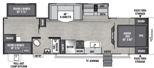
31 SE EXTERIOR LENGTH 35' 6"
