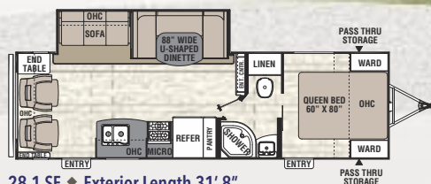
28.1 SE ♦ Exterior Length 31' 8"
